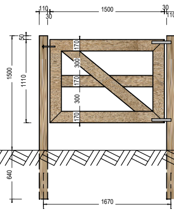
Typ 1500-3
