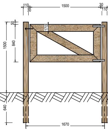
Typ 1500-2
