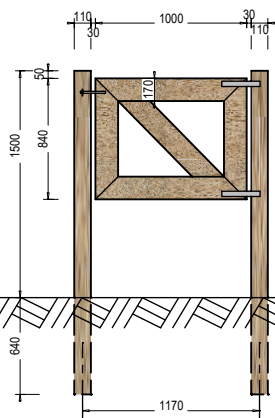
Typ 1500-2
