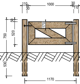
Typ 750-2
