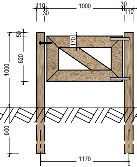
Typ 1000-1/2
