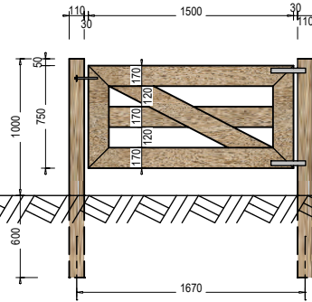
Typ 1000-3
