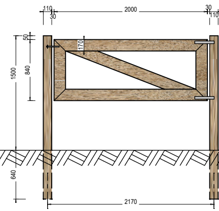
Typ 1500-2
