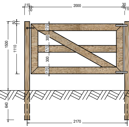
Typ 1500-3
