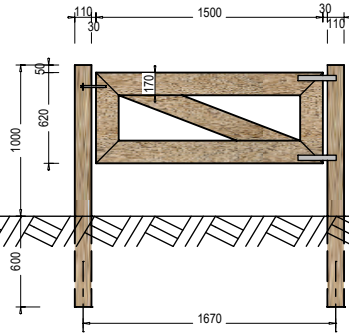
Typ 1000-1/2
