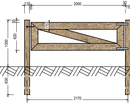
Typ 1000-2
