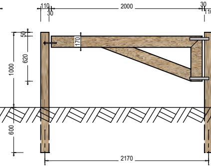
Typ 1000-1/2
